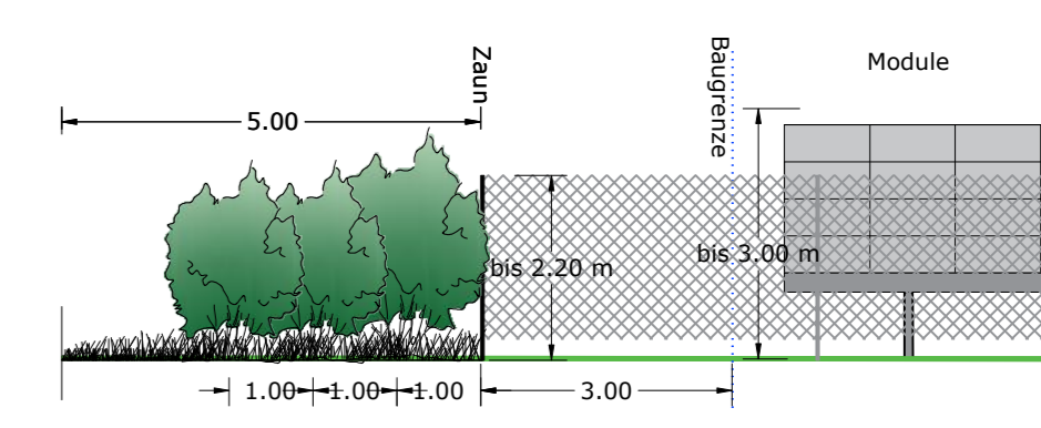
Systemschnitt Eingrünung, M 1: 100
